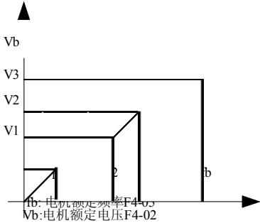
图 5-5.V/F 曲线设定示意图
