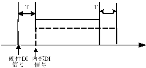
图 4-27.X(DI)延迟设置
