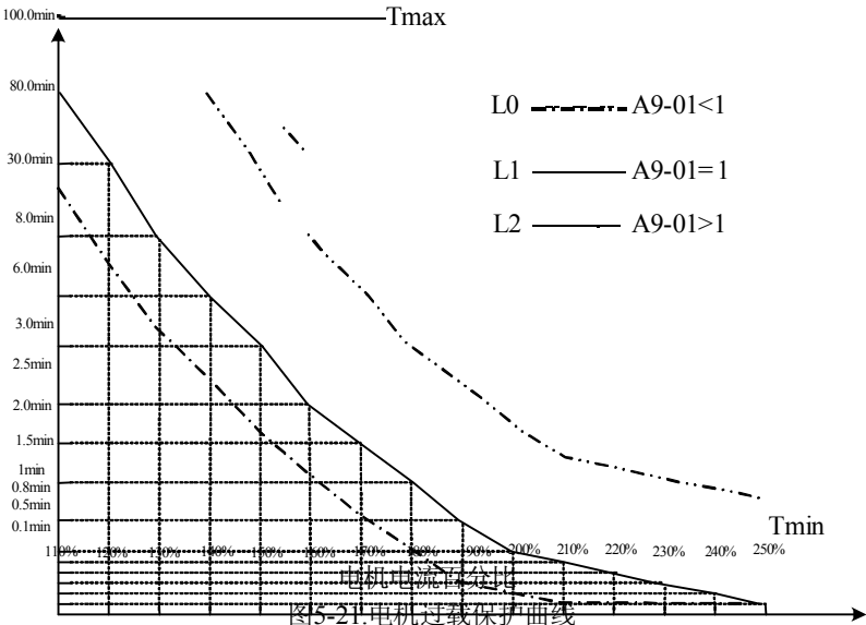
图5-21 电机过载保护曲线
