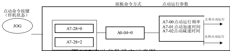
图4-15.点动参数设定示意图
