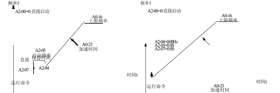
图4-11.直接启动示意图
