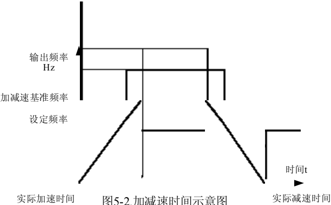
图5-2.加减速时间示意图
