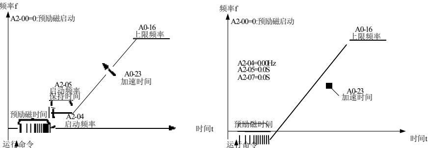
图4-12.预励磁启动示意图
