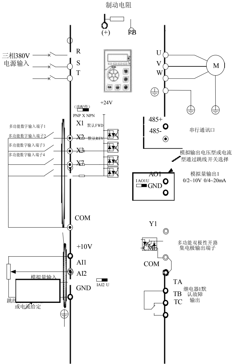
图3-6.2.2kW（4T:380V 2.2 kW）以下三相变频器接线图
