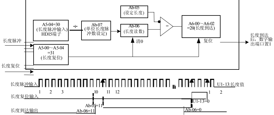
图 4-23.定长控制模式功能码设置
