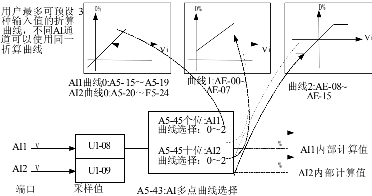
图 4-28.AI 信号对应实际给定
