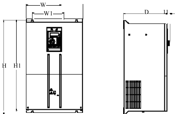
图 2-5. 11~132KW 钣金机箱外形尺寸及安装尺寸示意图
