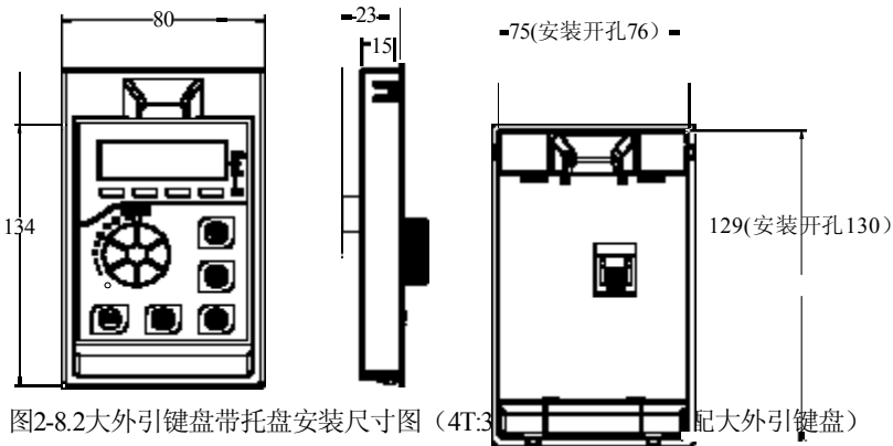
图2-8.1小外引键盘带托盘安装尺寸图 (4T:380V, 7kW以下标配小外引键盘)
