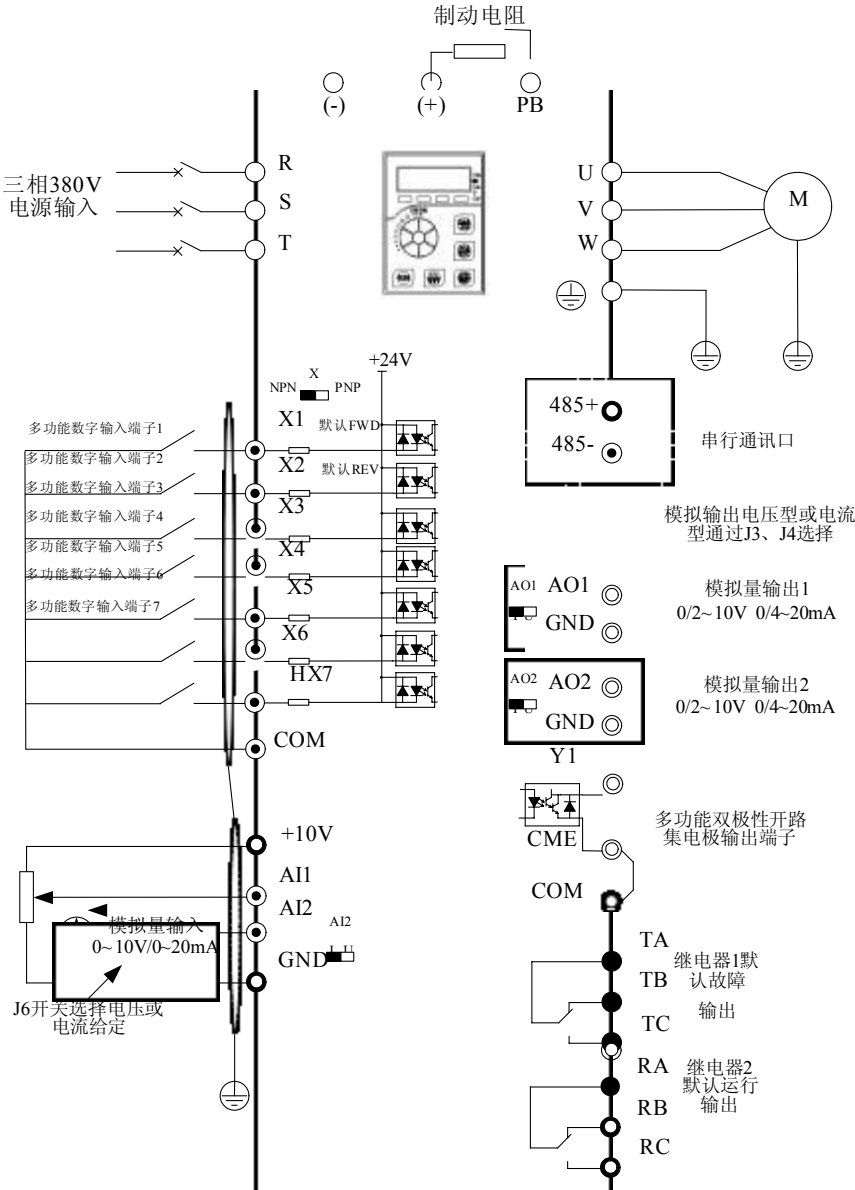
图 3-7. 4.0~22kW (4T:380V 4.0 ~ 22kW) 三相变频器接线图 备注：数字输入端子 X 跳线开关出厂默认 NPN 模式（即 X 短接 COM 有效），AI2,AO1,AO2 跳线开关出厂默认电压模式
