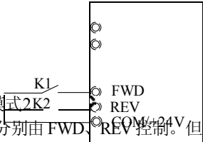
图5-8.两线式运转模式2
