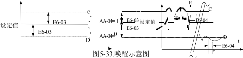
图5-33.唤醒示意图
