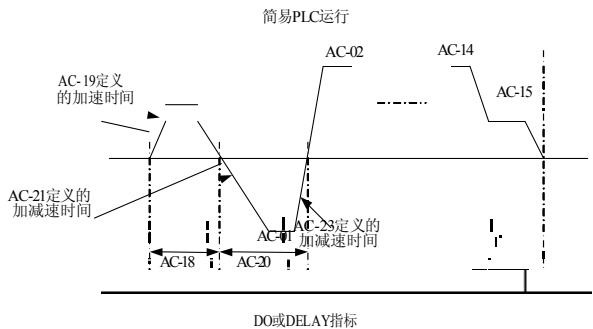
图5-29 简易PLC示意图
