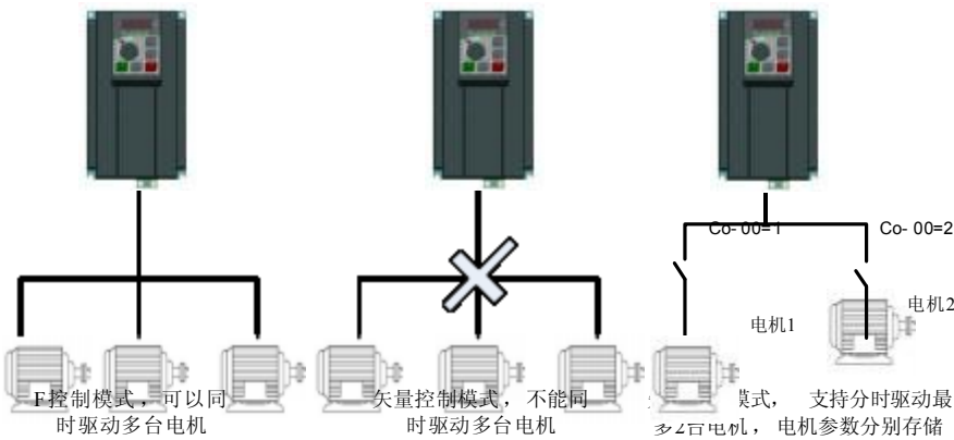
图 4-26.多组电机的切换
