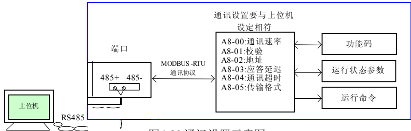
图4-30.通讯设置示意图
