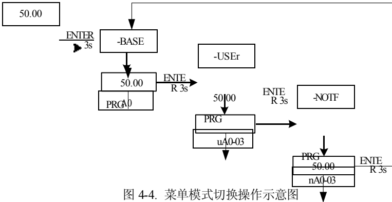
图 4-4. 菜单模式切换操作示意图
