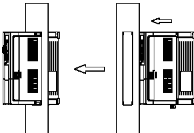
图3-3.CT500/CT500S变频器塑胶结构穿墙式安装图
