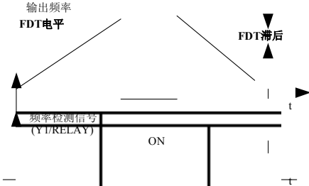
图 5-15.FDT 电平示意图
