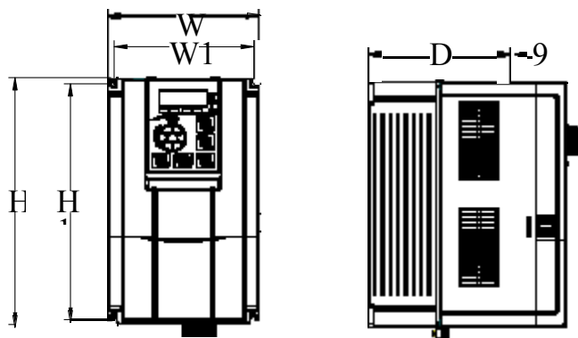
图 2-4. 7.5KW 以下塑胶外形尺寸及安装尺寸示意图
