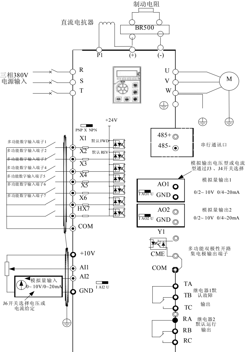
图3-9. 75Kw（4T-380V 75 Kw）及以上三相变频器
