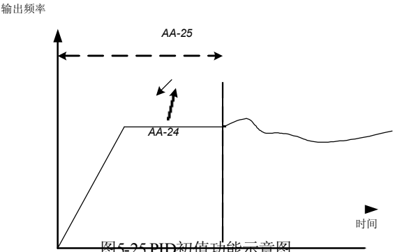
图5-25.PID初值功能示意图
