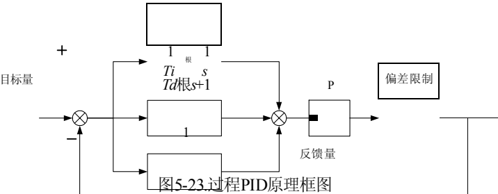
图5-23 过程PID原理框图
